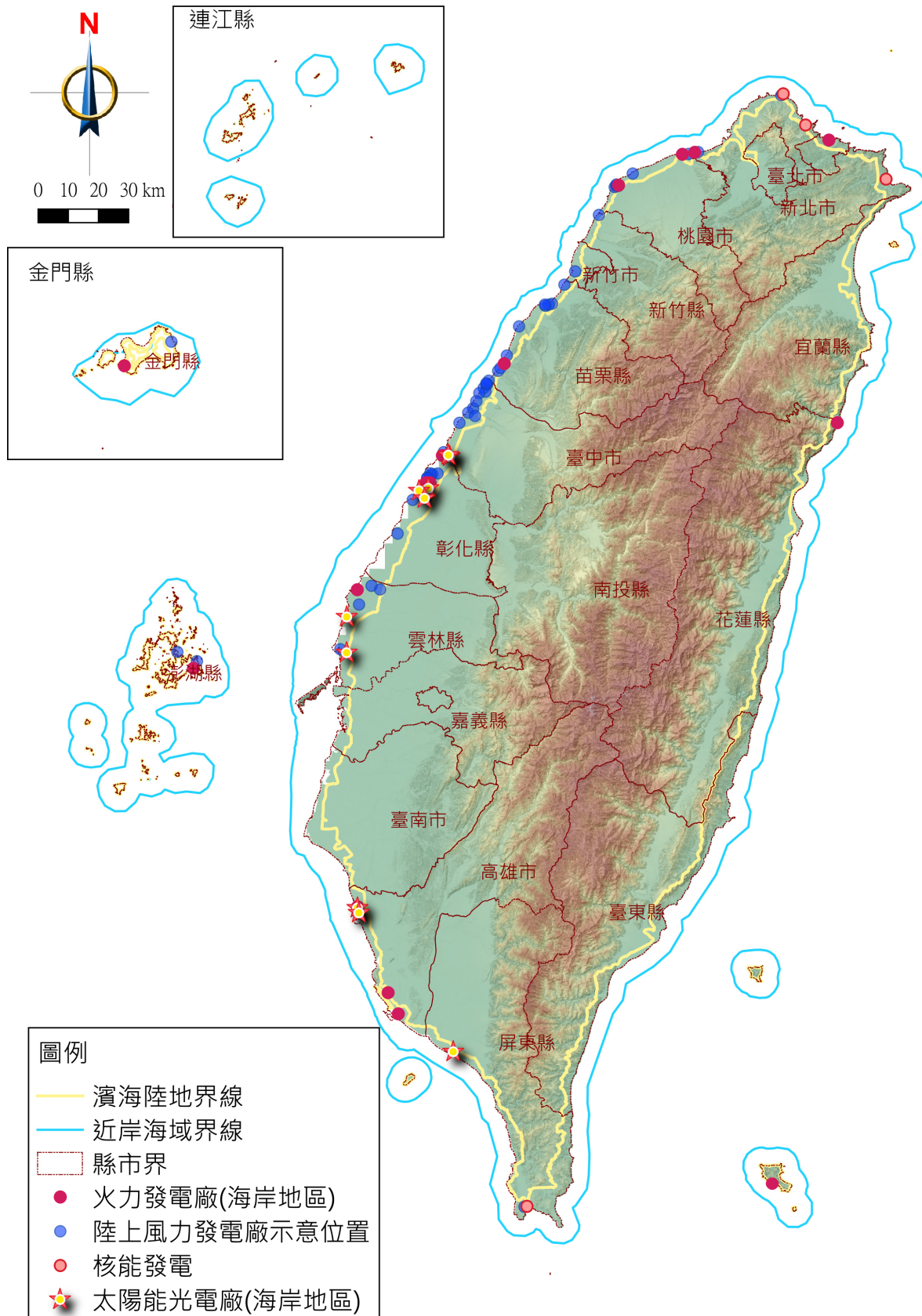
圖 2.3-1 海岸地區發電廠分布圖
