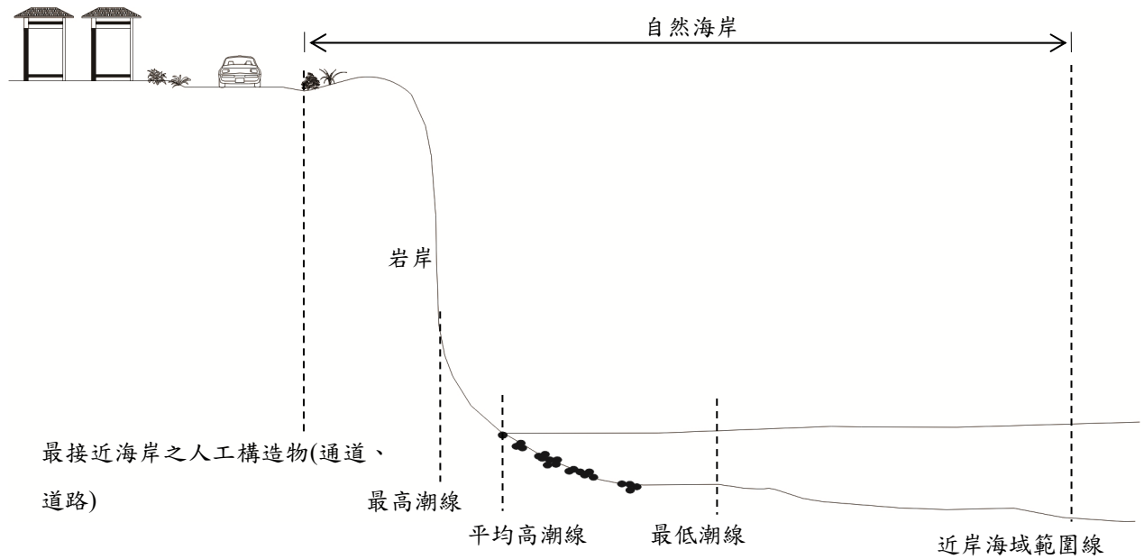
圖 2.3-7 自然海岸剖面示意圖 (B)
