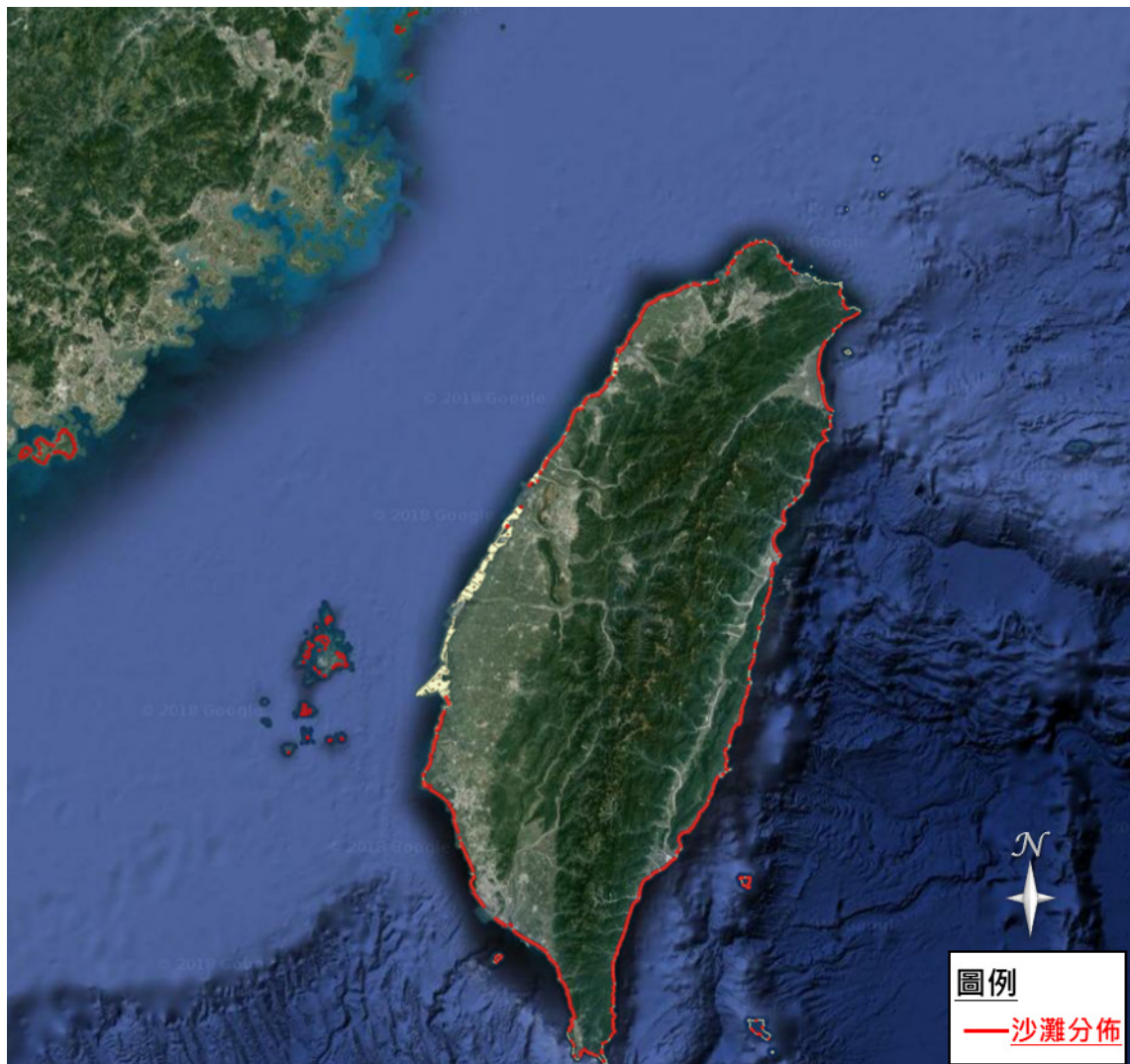
圖 2.3-10 臺灣及離島沙灘分佈現況圖
