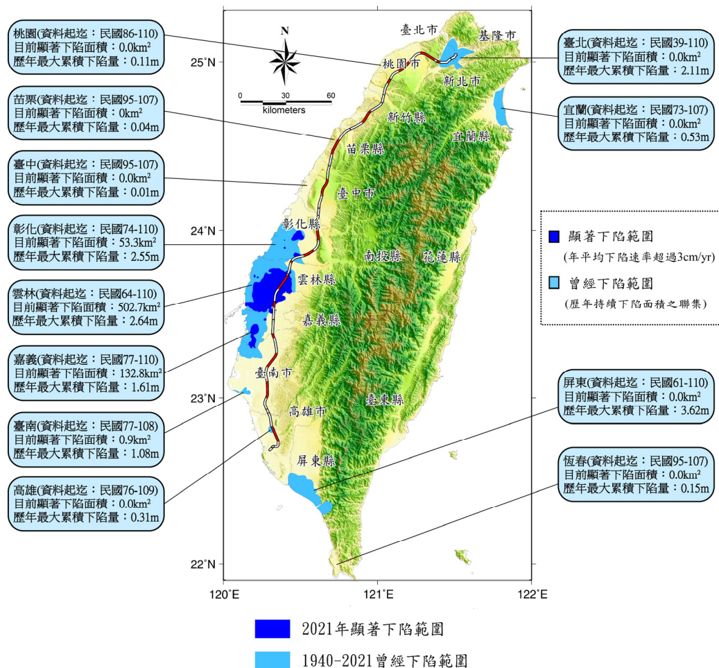
圖 2.2-2 臺灣地區地層下陷狀況說明圖
